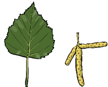
Bouleau pendant
