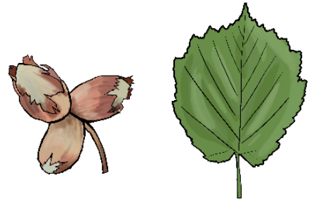
Noisetier
